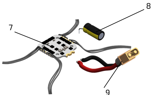
Kondensatorius (8) ir Maitinimo laidai (9) Greičio Regulatoriui (7)
