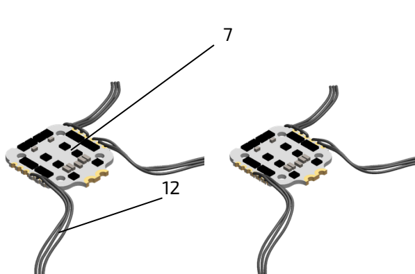
3-iojo variklio laidų litavimas
