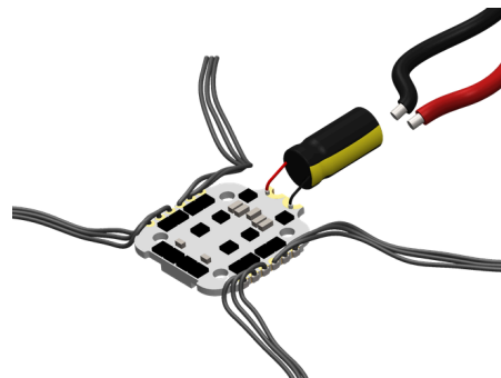
Kondensatoriaus (8) prilitavimas prie Greičio Regulatoriaus (7)
